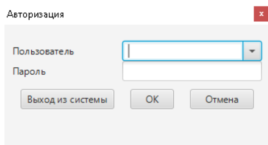
Рисунок 16. Функция logIn()
