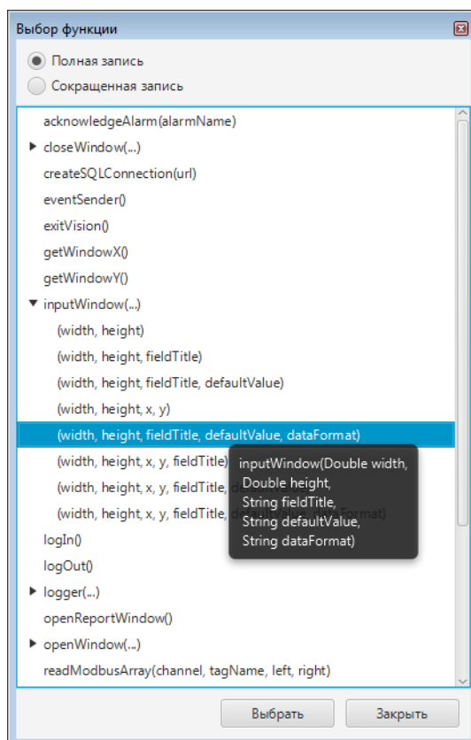
Рисунок 6. Всплывающая подсказка
