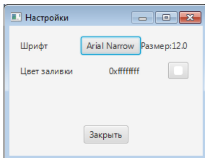
Рисунок 3. Кнопка "Настройки"
