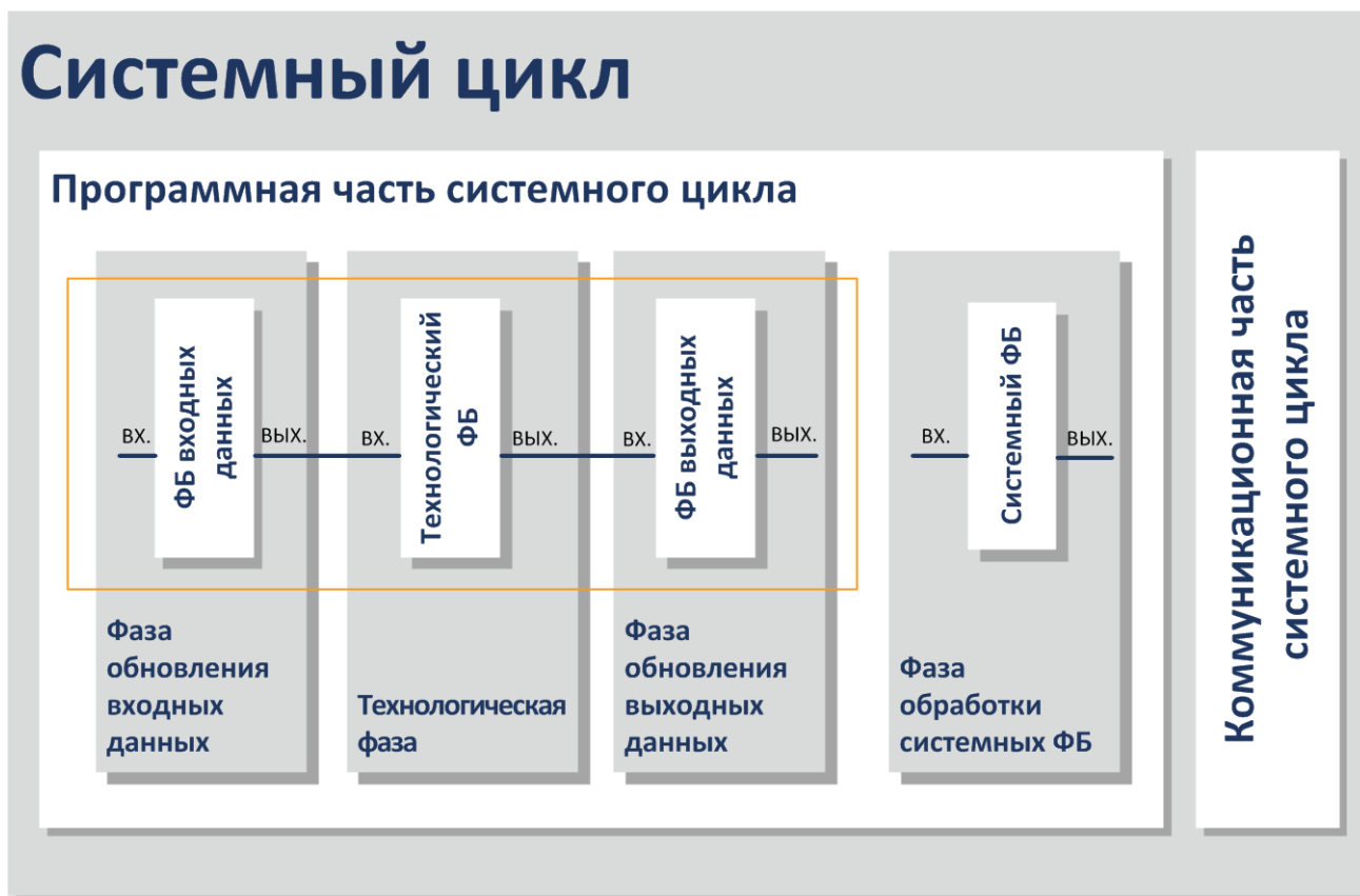
Рисунок 3. Системный цикл
