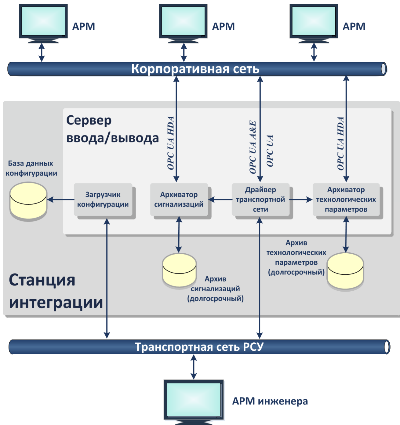
Рисунок 5. Станция интеграции
