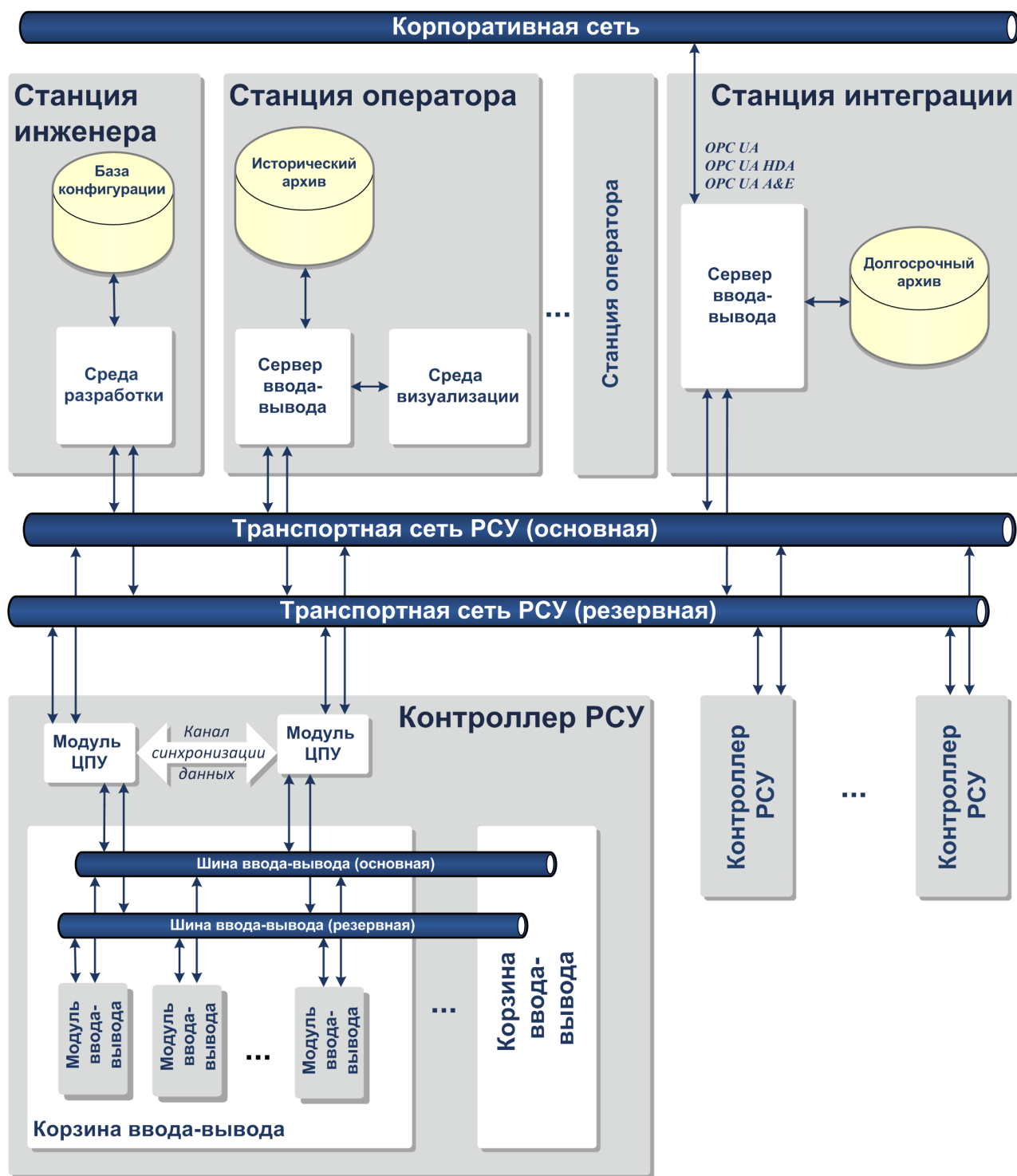
Рисунок 1. Пример структуры системы автоматизации на базе PCY
