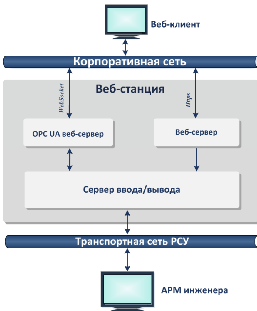
Рисунок 7. Веб-станция
