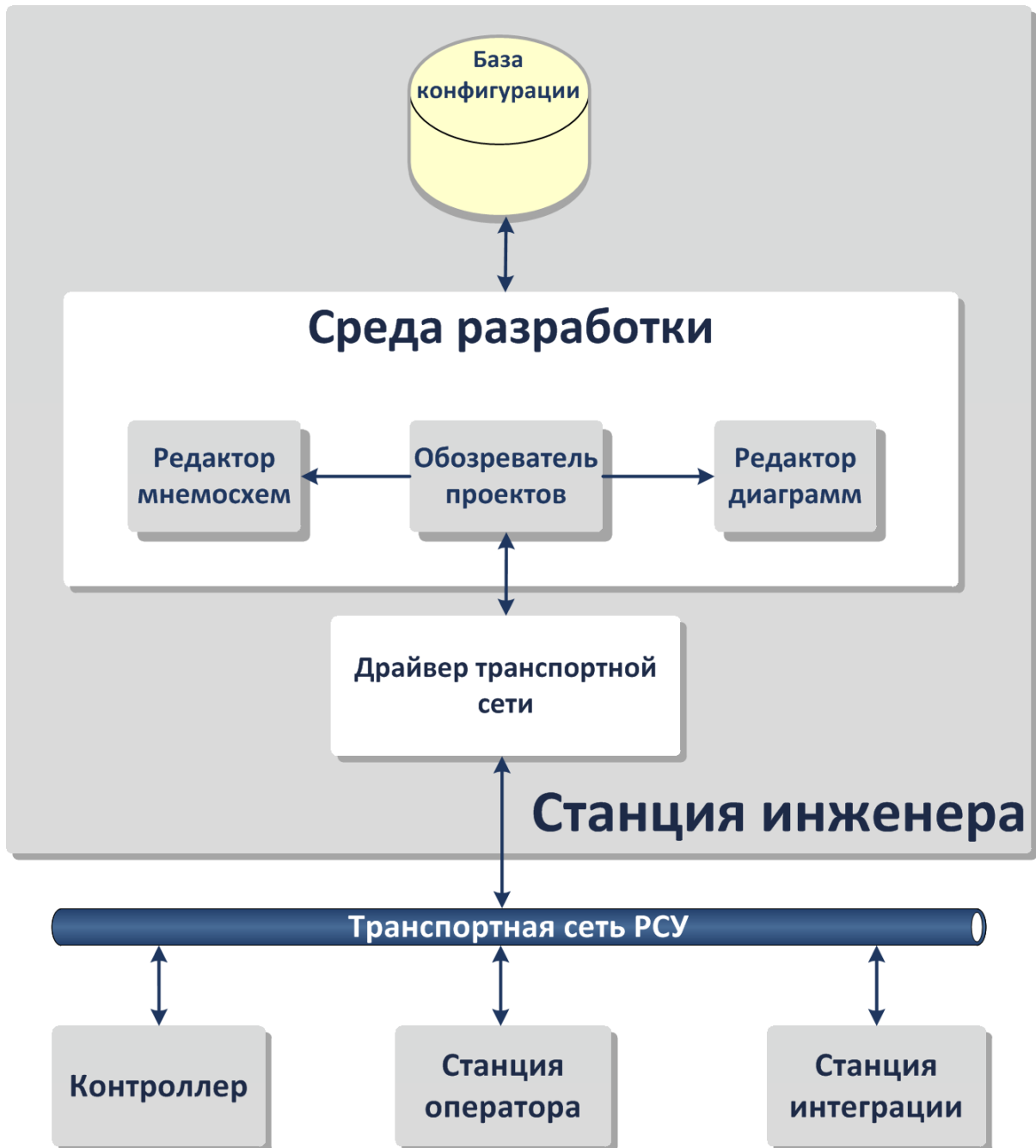
Рисунок 6. Станция инженера
