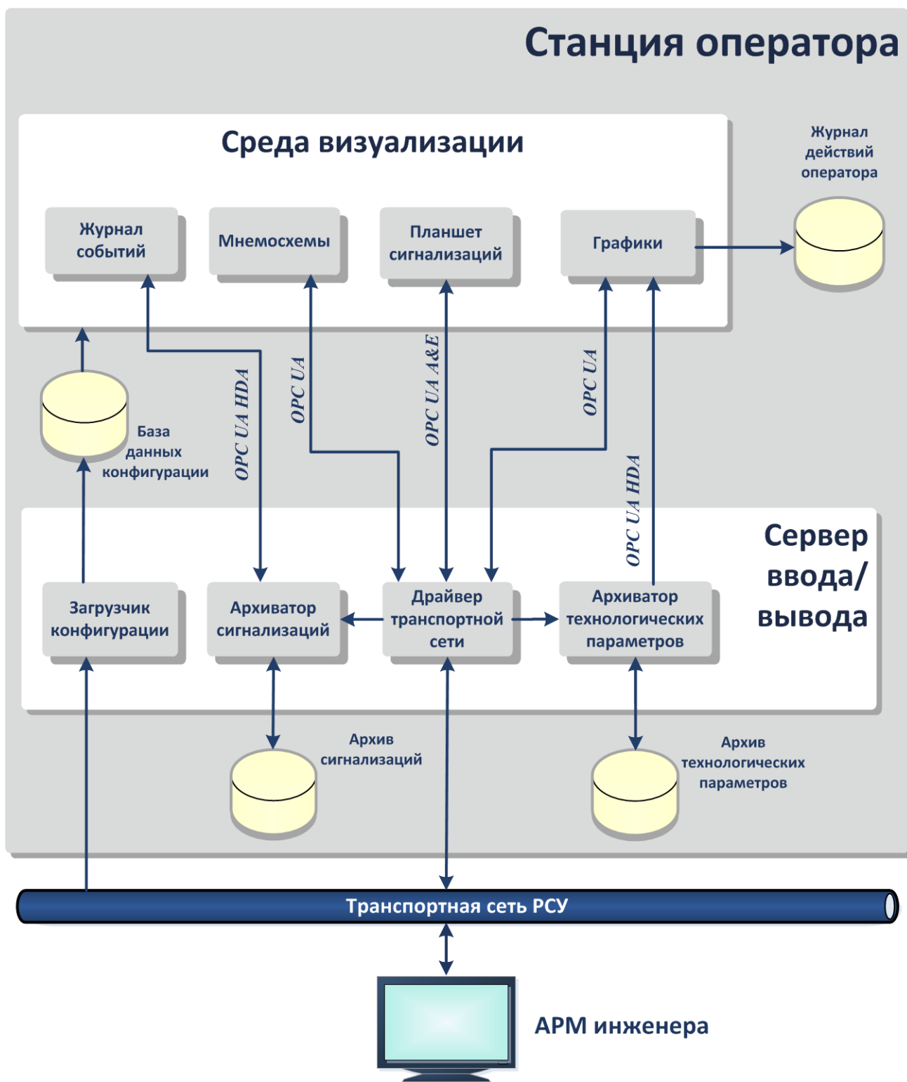
Рисунок 4. Станция оператора
