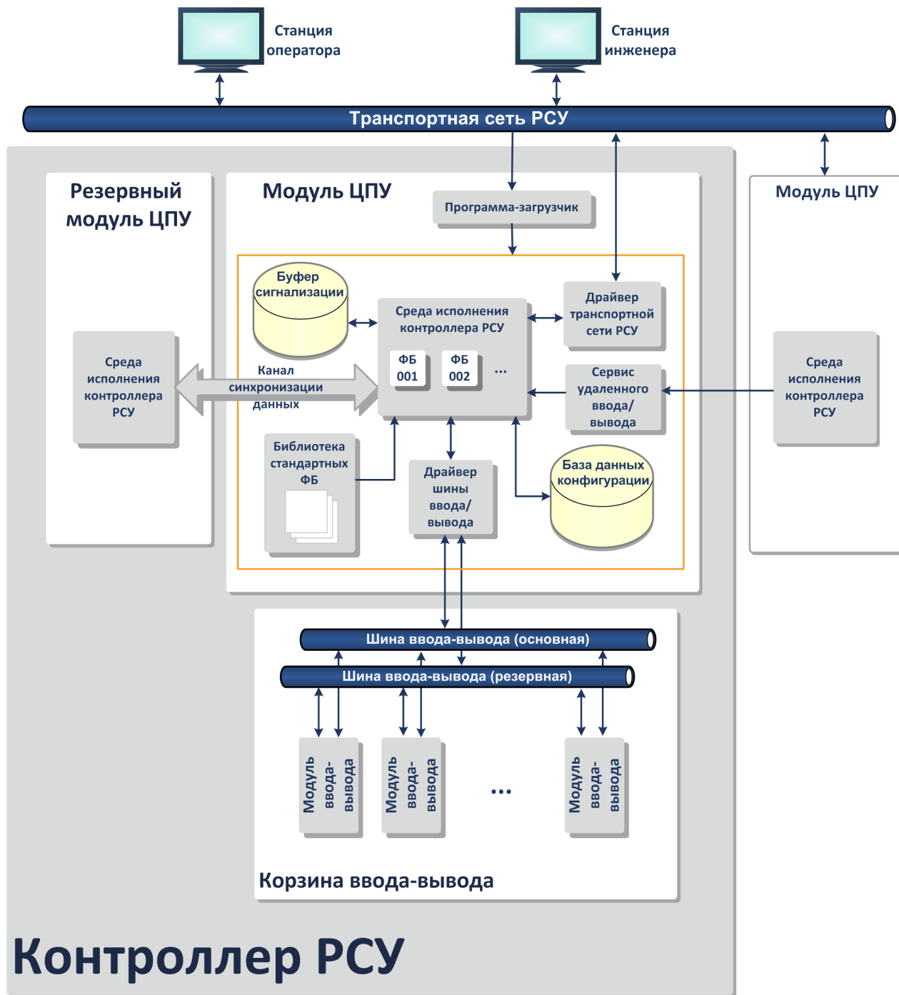
Рисунок 2. Структурная схема контроллера РСУ
