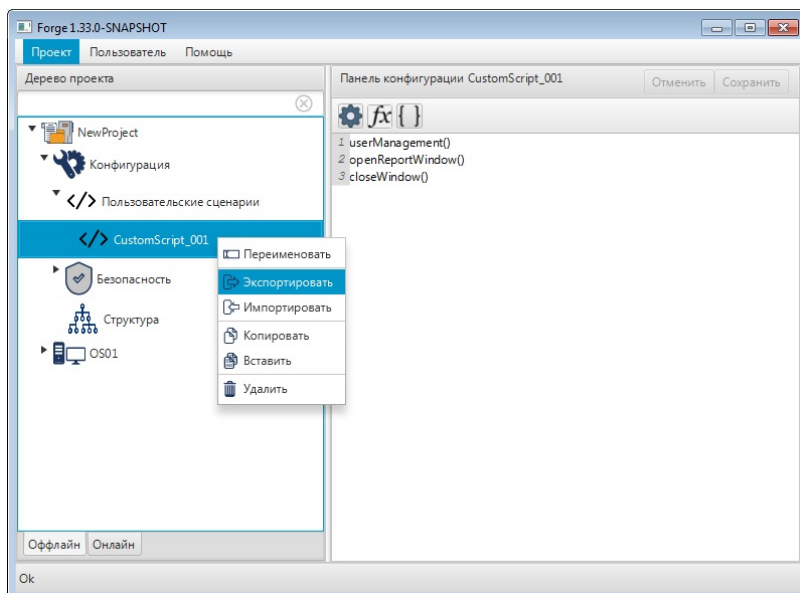
Рисунок 13. Экспорт пользовательского сценария
