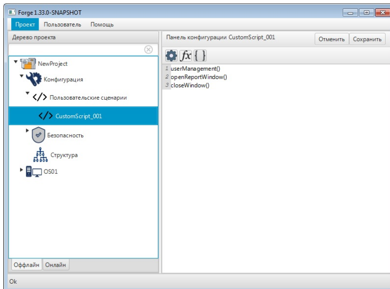
Рисунок 8. Окно конфигурации пользовательского сценария
