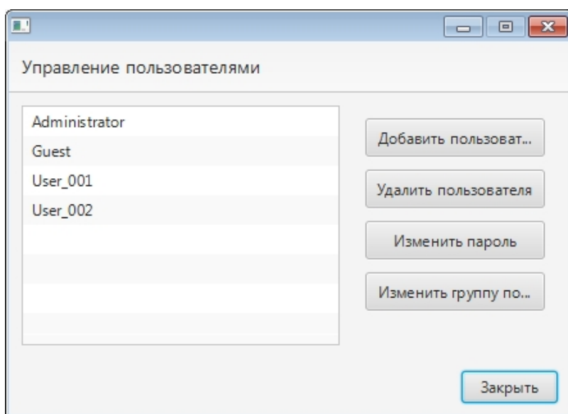
Рисунок 17. Функция userManagement()
