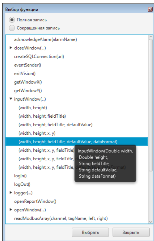
Рисунок 6. Всплывающая подсказка
