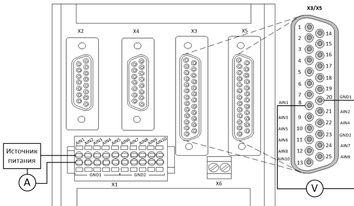
Рисунок 1 – Схема подключения средств поверки к ПТН-Е2Н-01 при опробовании
