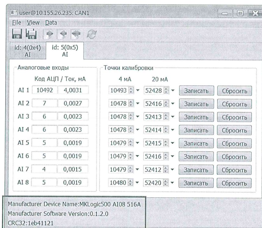
Рисунок 2. Окно калибровки в ПО «Калибратор МКLogic-500» для модулей аналогового ввода.
