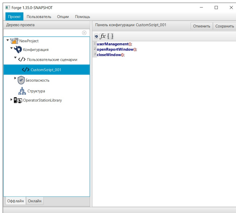
Рисунок 8. Окно конфигурации пользовательского сценария
