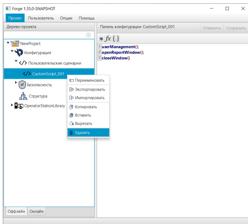
Рисунок 15. Удаление пользовательского сценария
