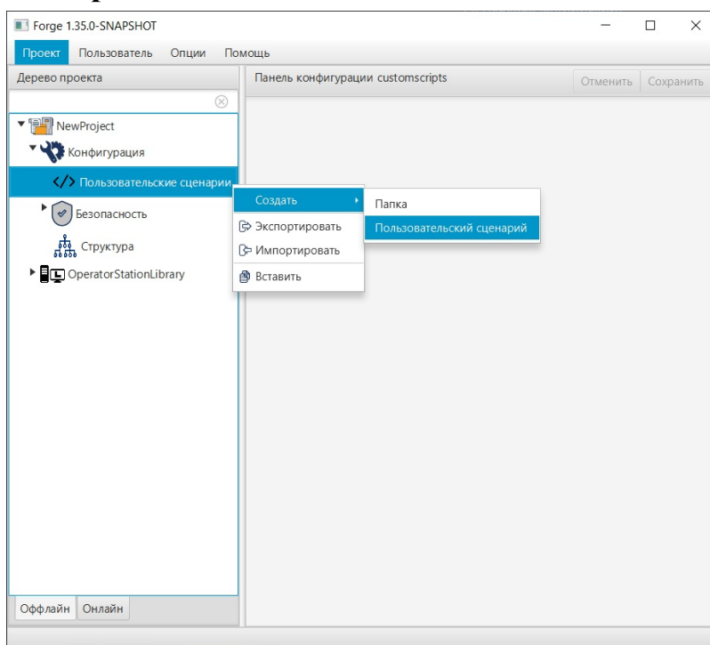
Рисунок 1. Создание пользовательского сценария
